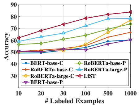
(b) RTE
